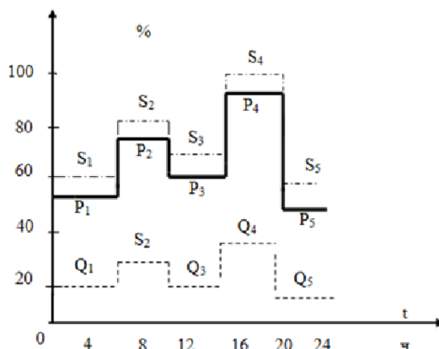
Рисунок - Суточные графики активной, реактивной и полной мощности Задание 7
