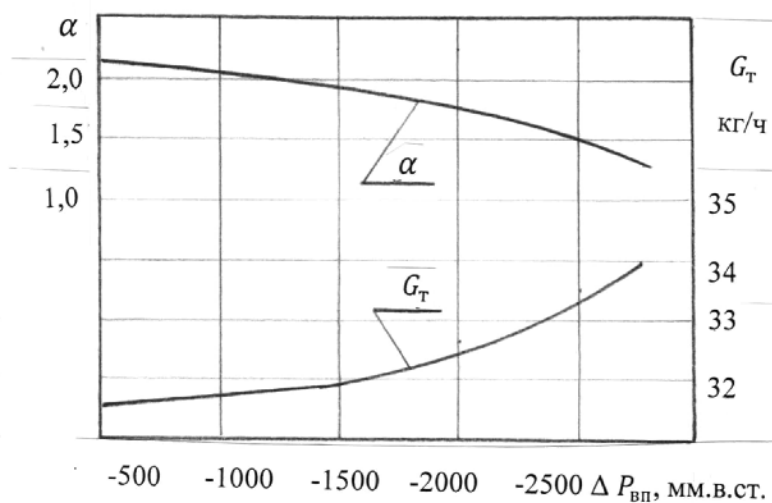
Характеристика по разряжению на впуске
