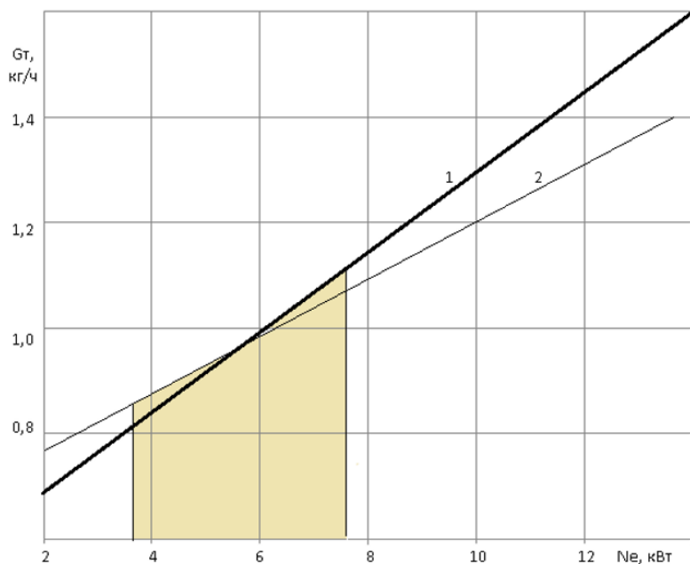
Относительная экономичность двигателей малой мощности 1 – бензиновые, 2 - дизельные
