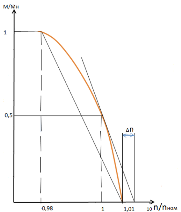
Регуляторная характеристика дизеля
